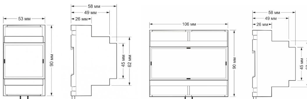
Габаритные размеры SH-DOI3.10SMS1 и SH-DOI6.10SMS1
