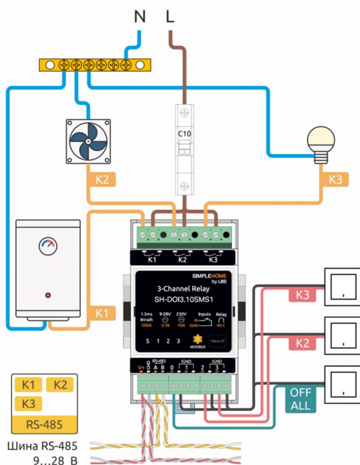
Пример схемы подключения SH-DOI3.10SMS1
